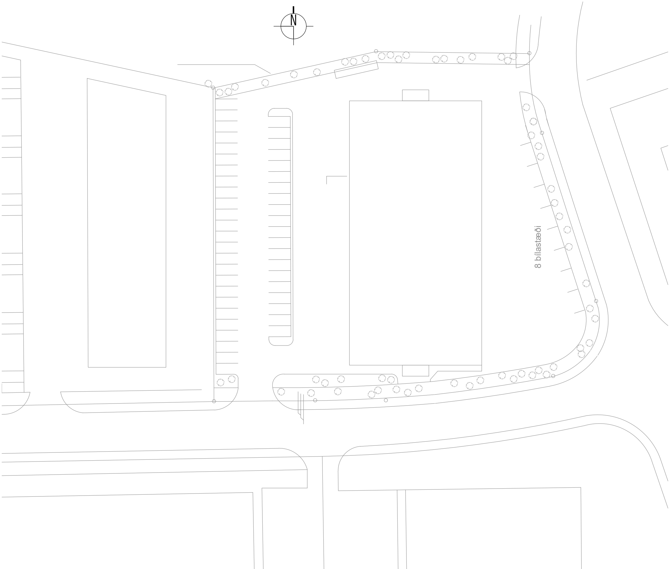
Afstöðumynd 1:500
